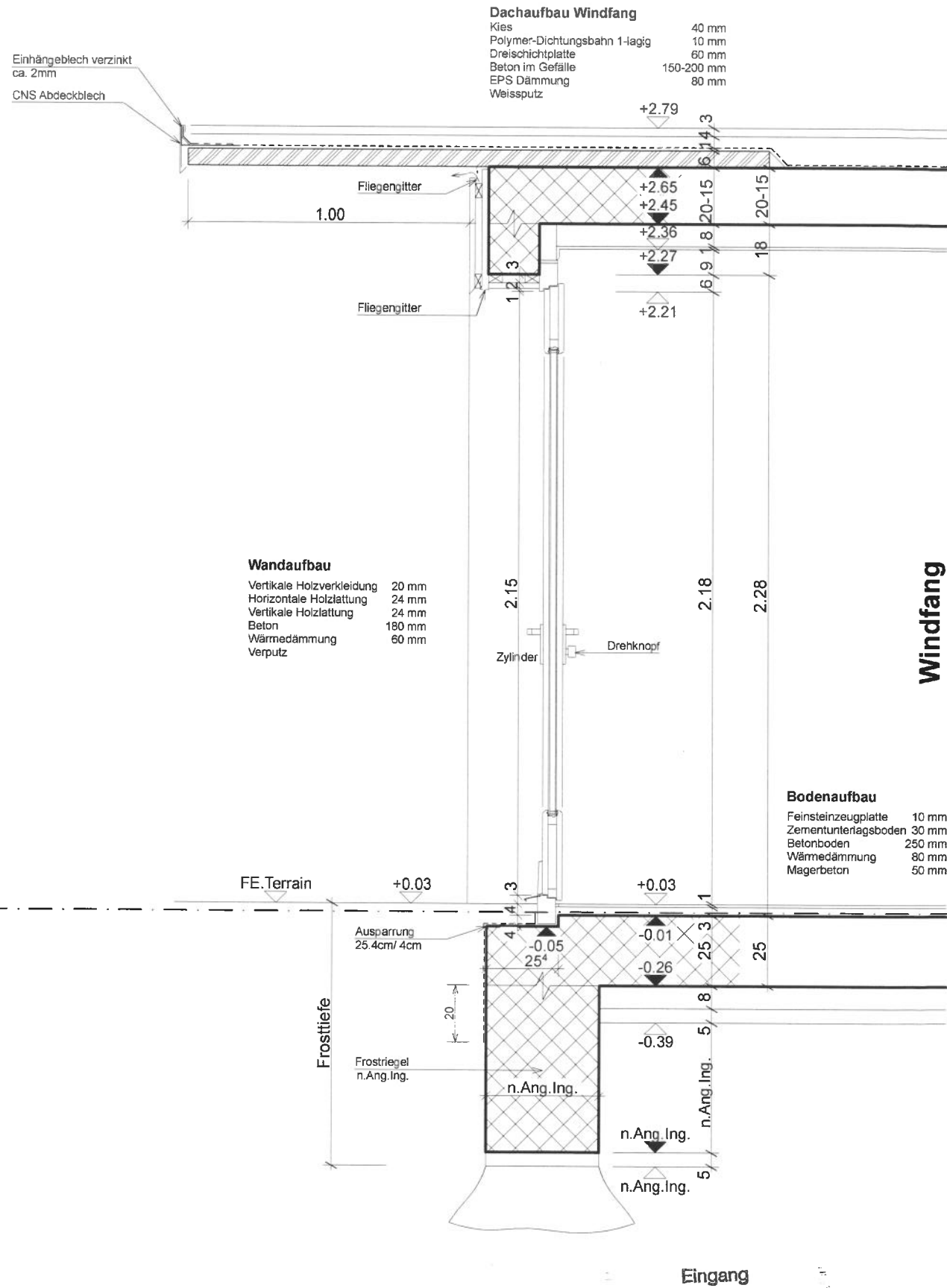
Schnitt 3 - 7. Dez. 2020
