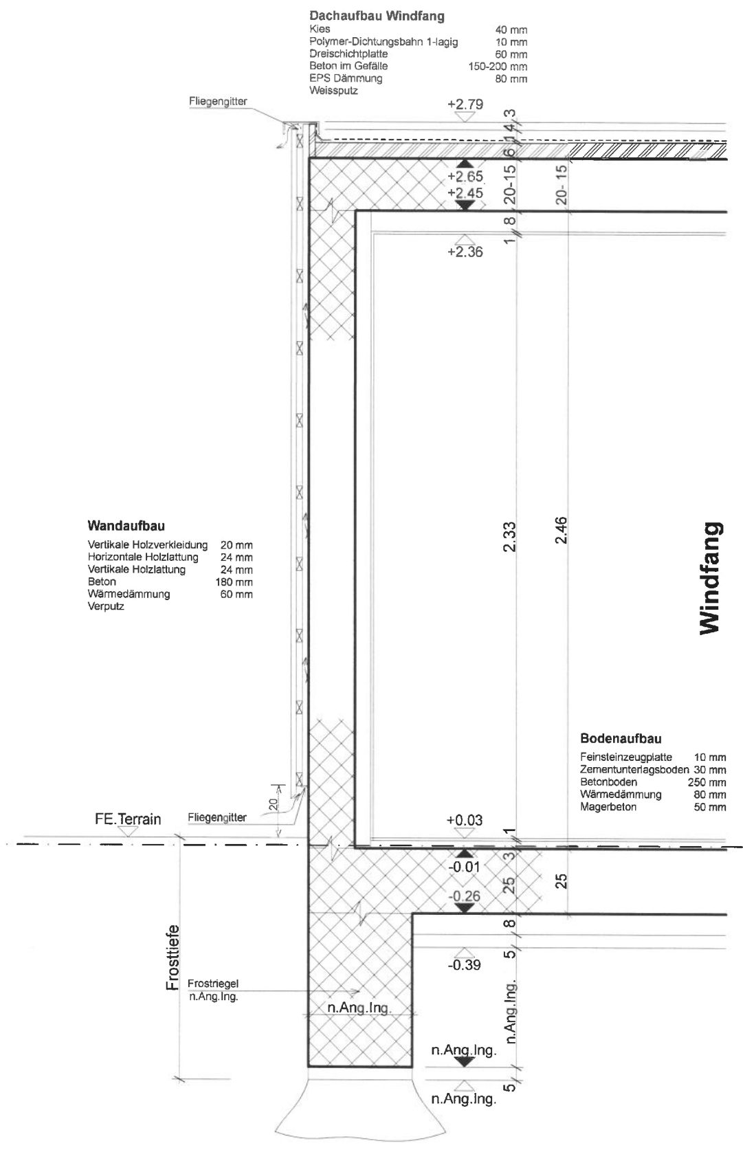
Schnitt 4
