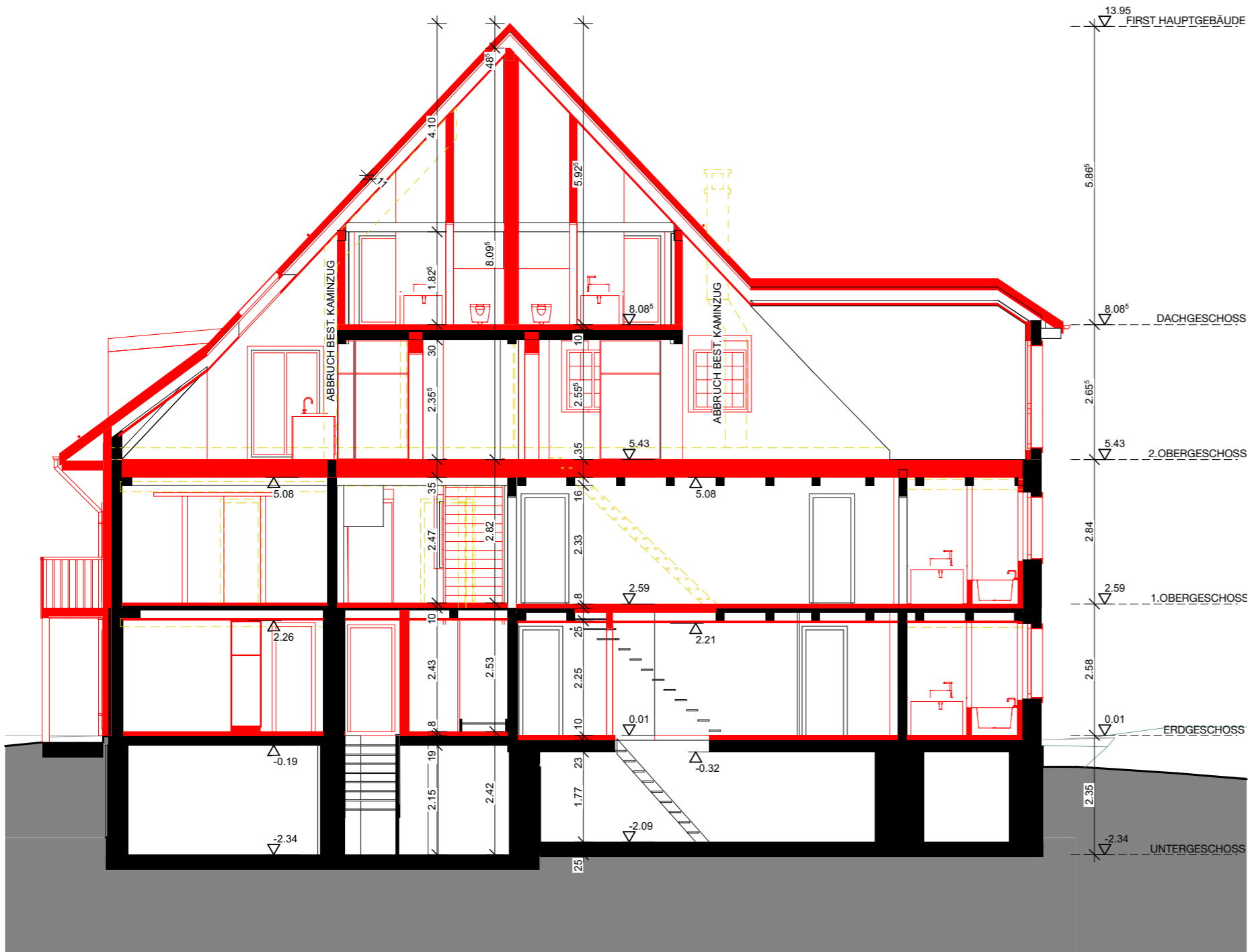
SCHNITT 02-02
