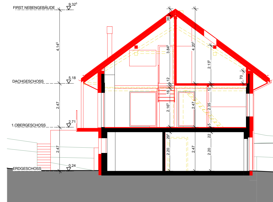
SCHNITT 03-03
