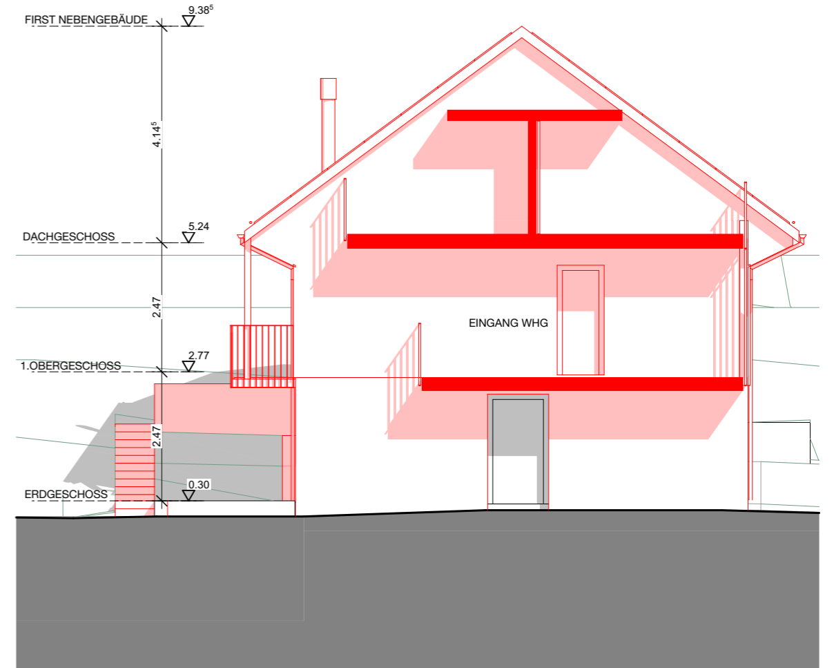
ANSICHT SÜD NEBENGEBÄUDE
