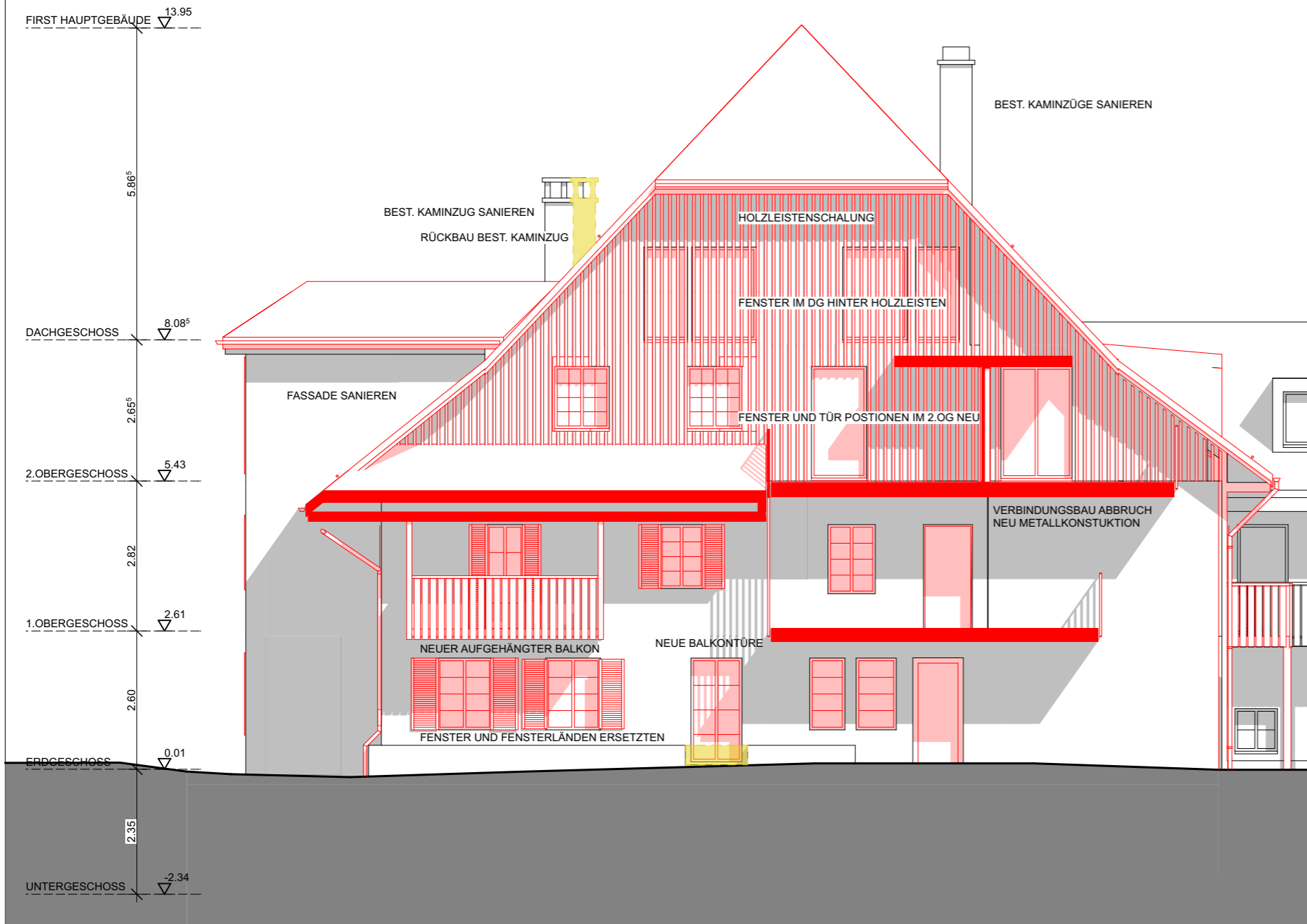
ANSICHT NORD HAUPTGEBÄUDE
