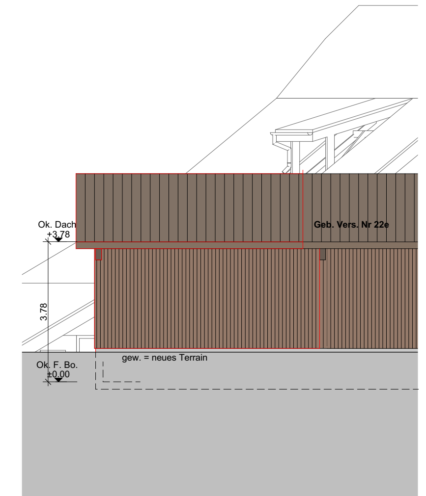
Westfassade
