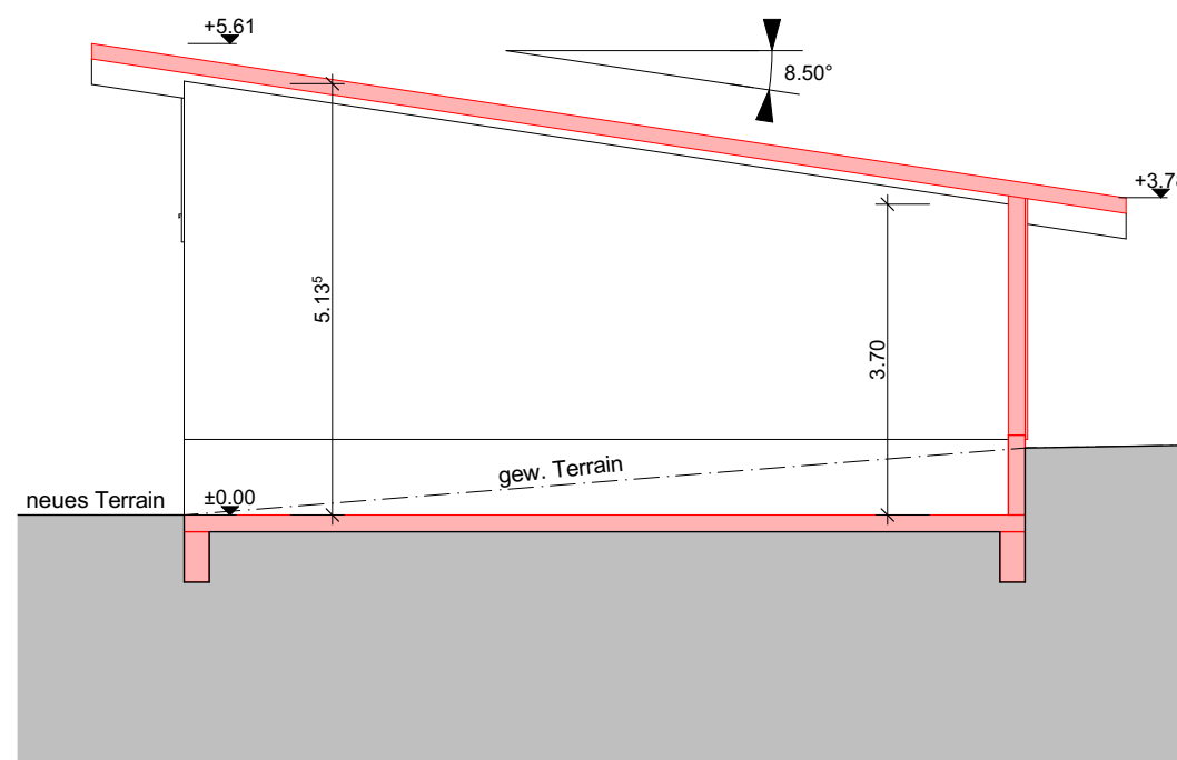
Schnitt C-C
