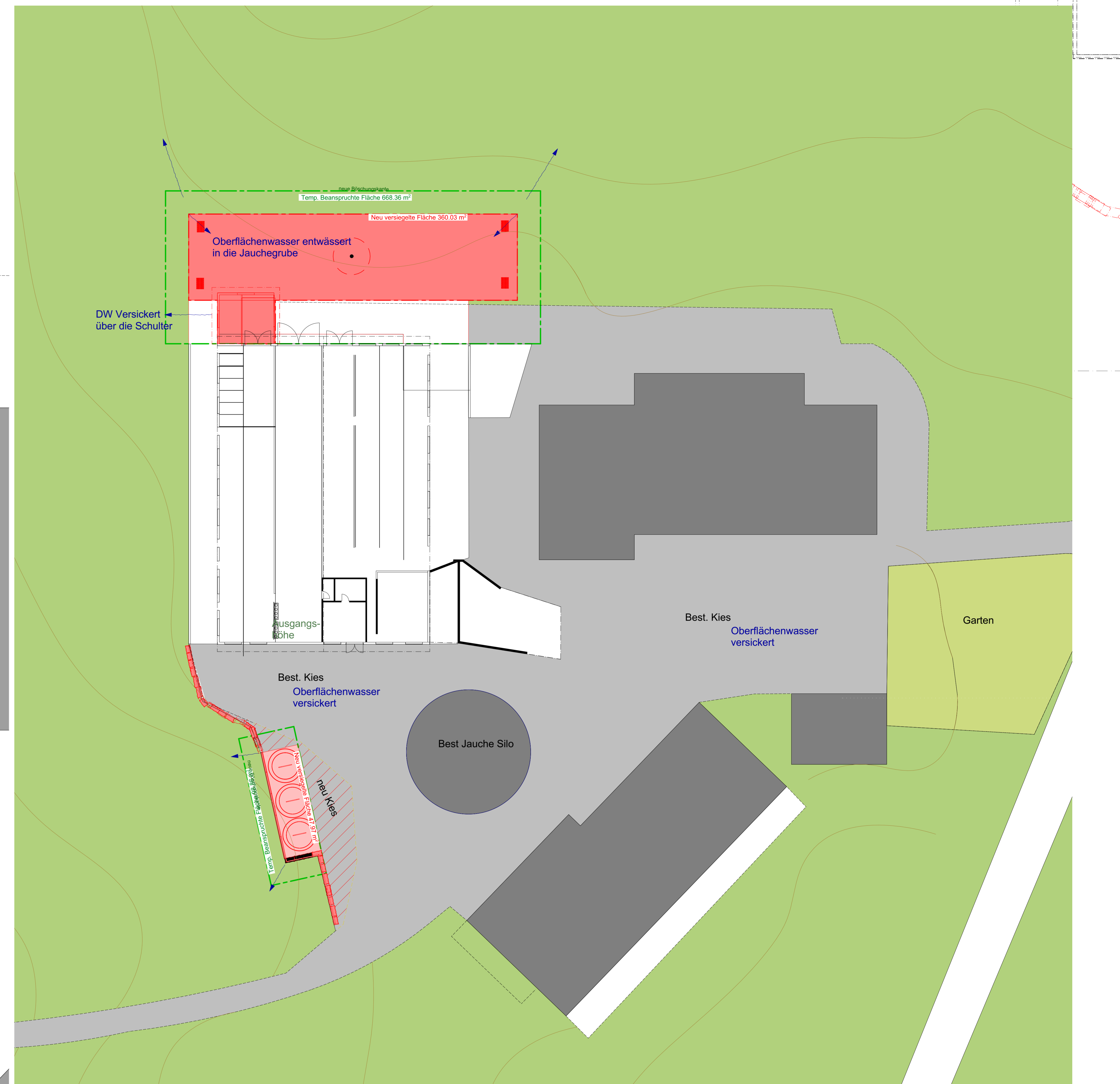
Übersichtsplan 1:200
