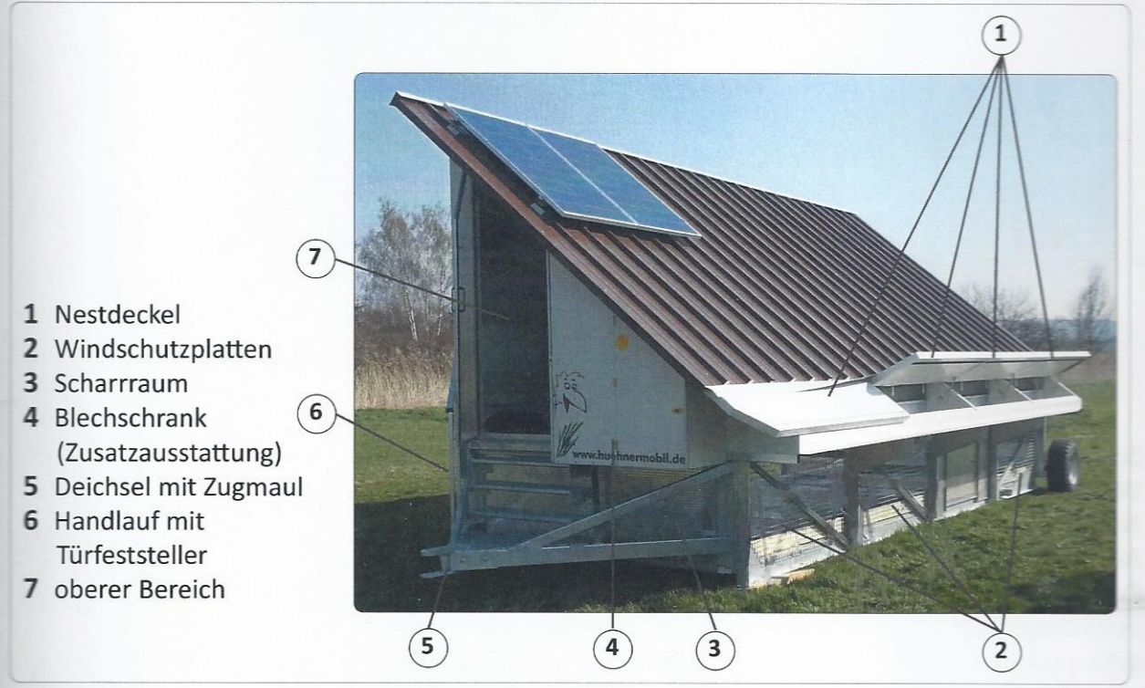
Bild 1: Frontansicht
