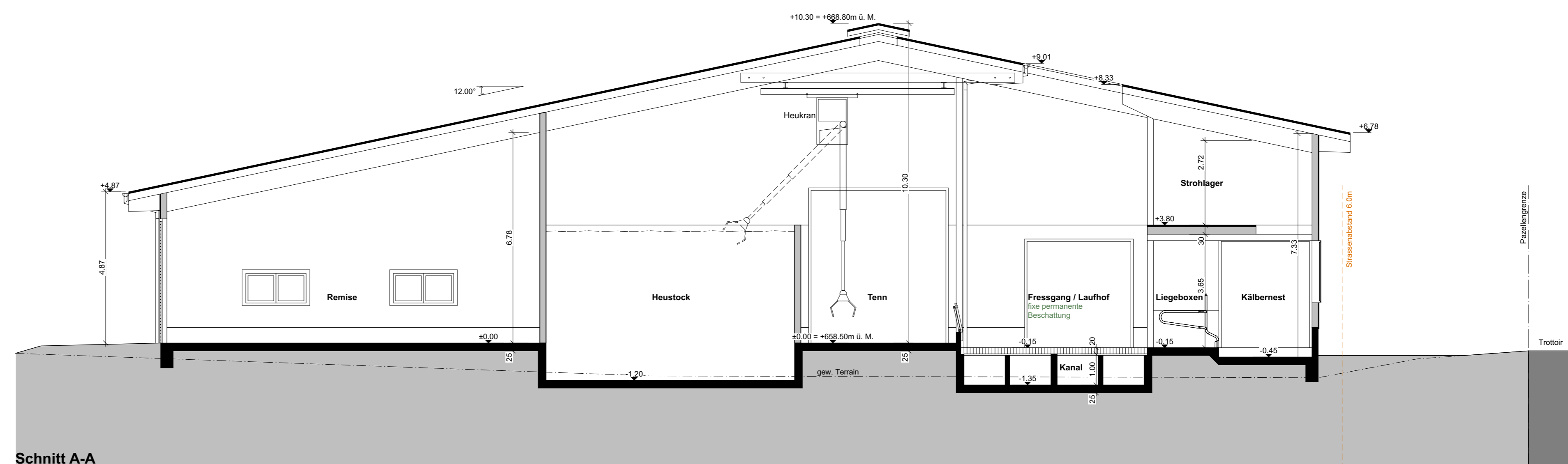
Schnitt A-A
