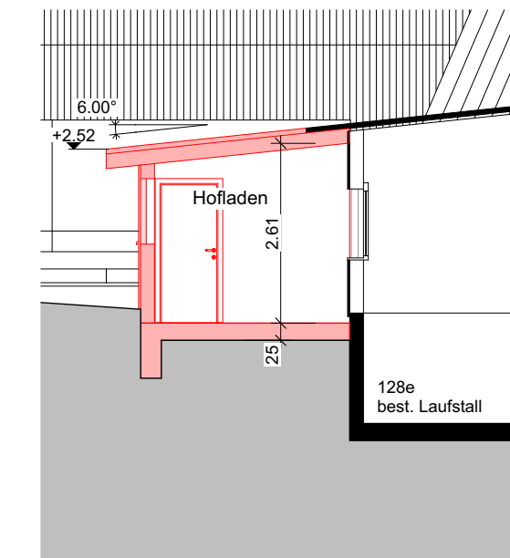
Schnitt A-A
