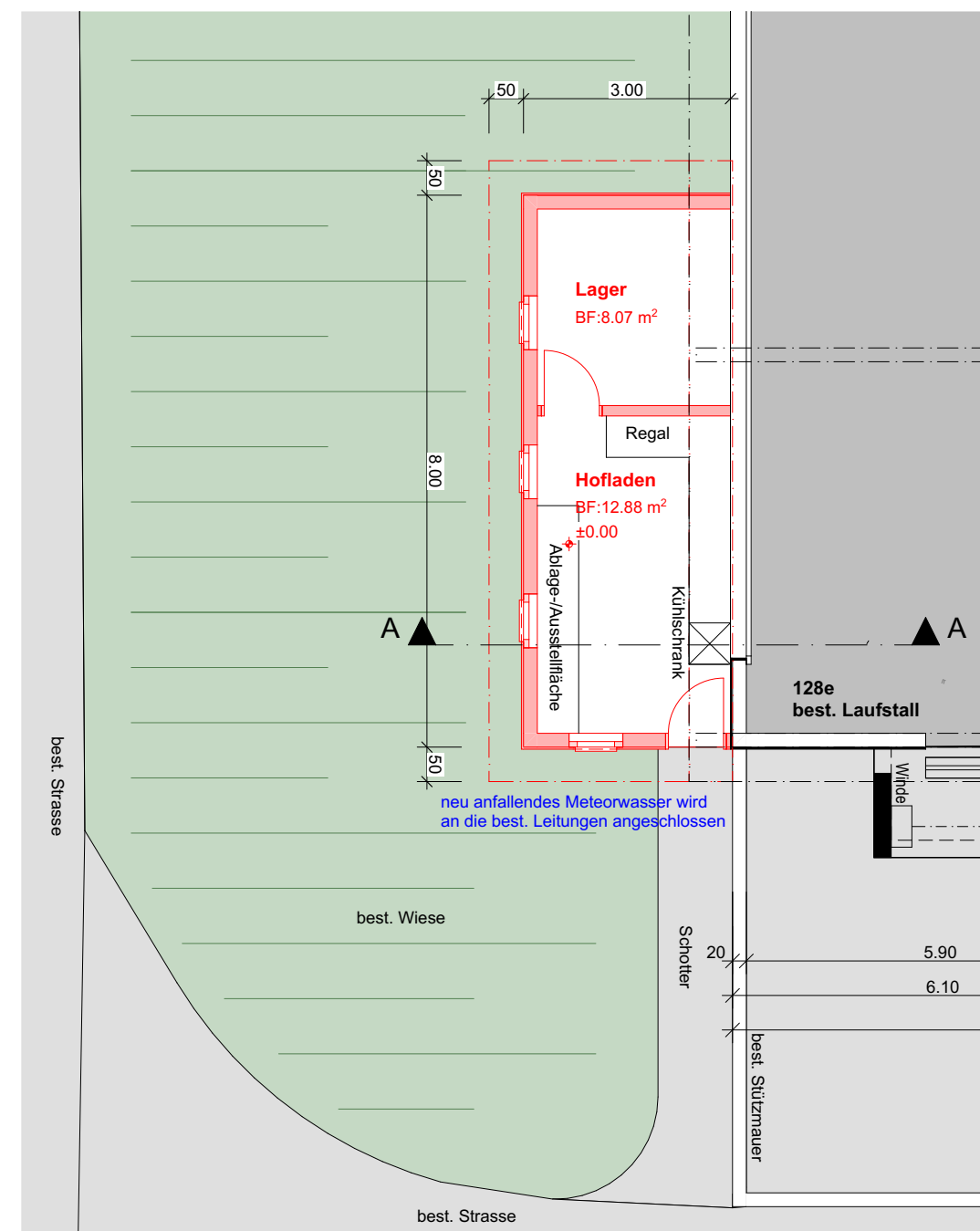
Erdgeschoss
