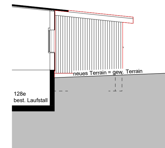
Nordwestfassade
