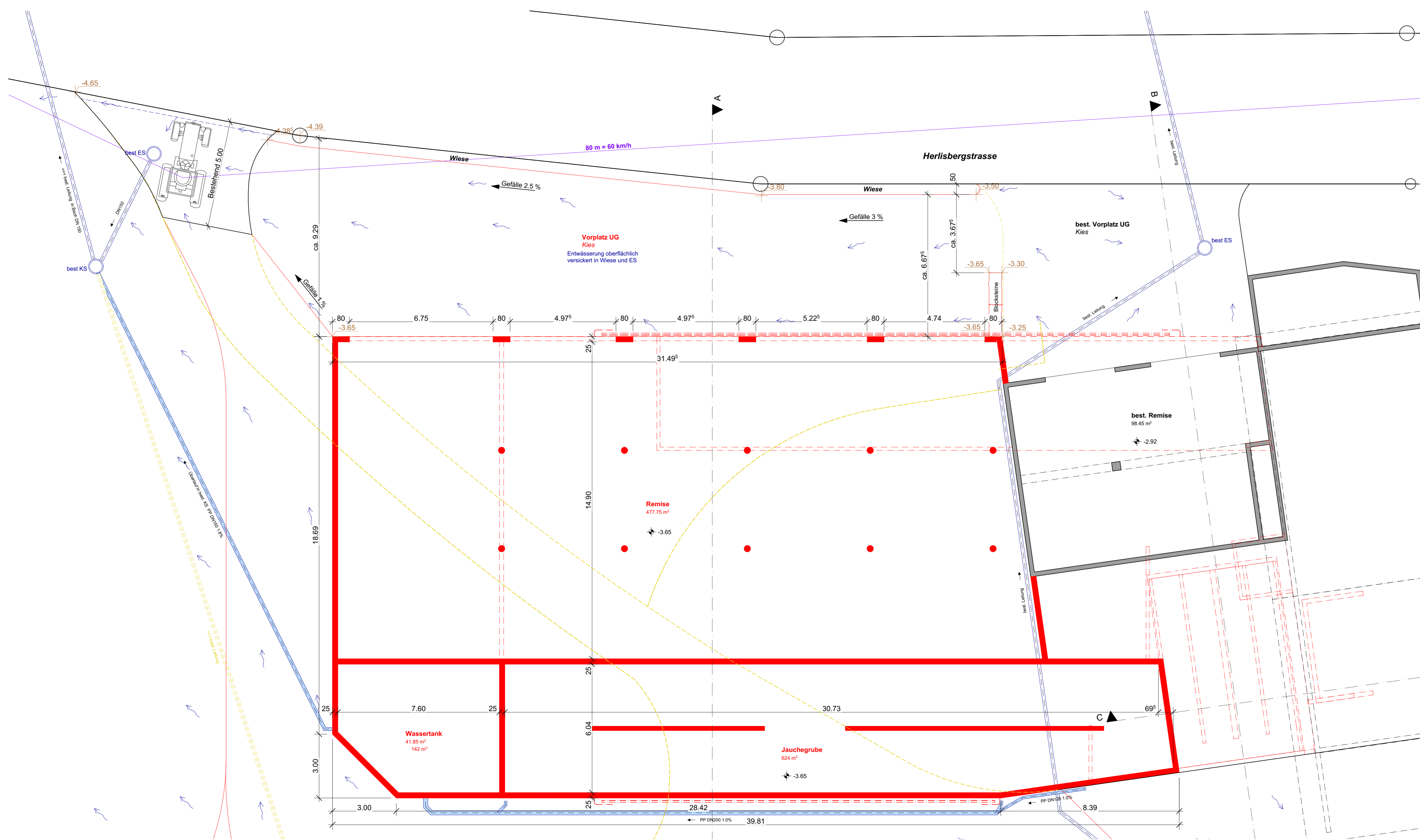
Untergeschoss 1:100
