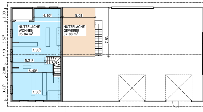
OBERGESCHOSS BESTAND
