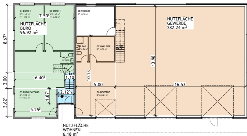
ERDGESCHOSS BESTAND
