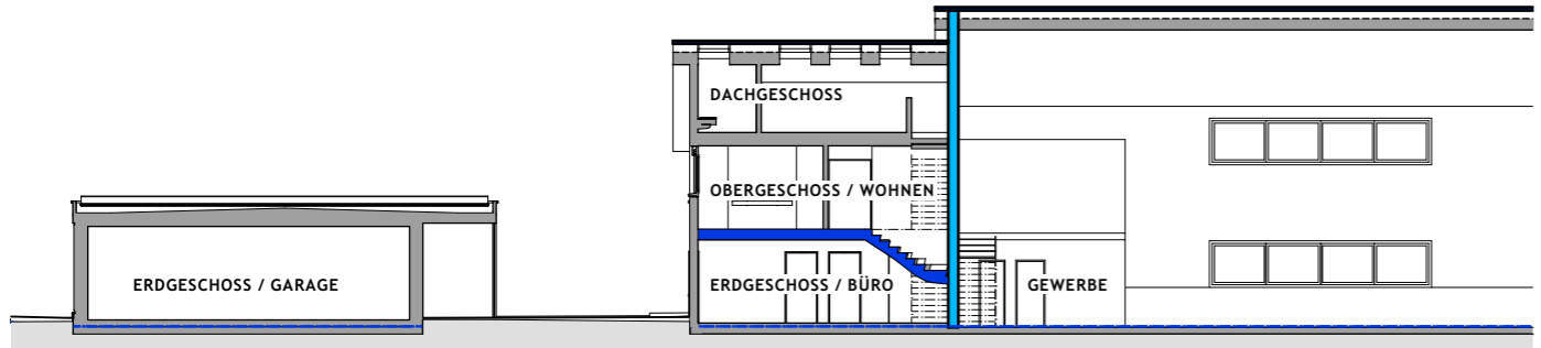
SCHNITT B-B
