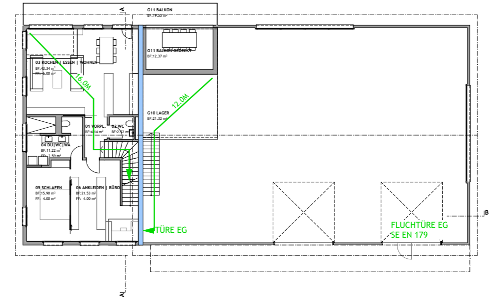
OBERGESCHOSS
