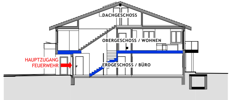
SCHNITT A-A
